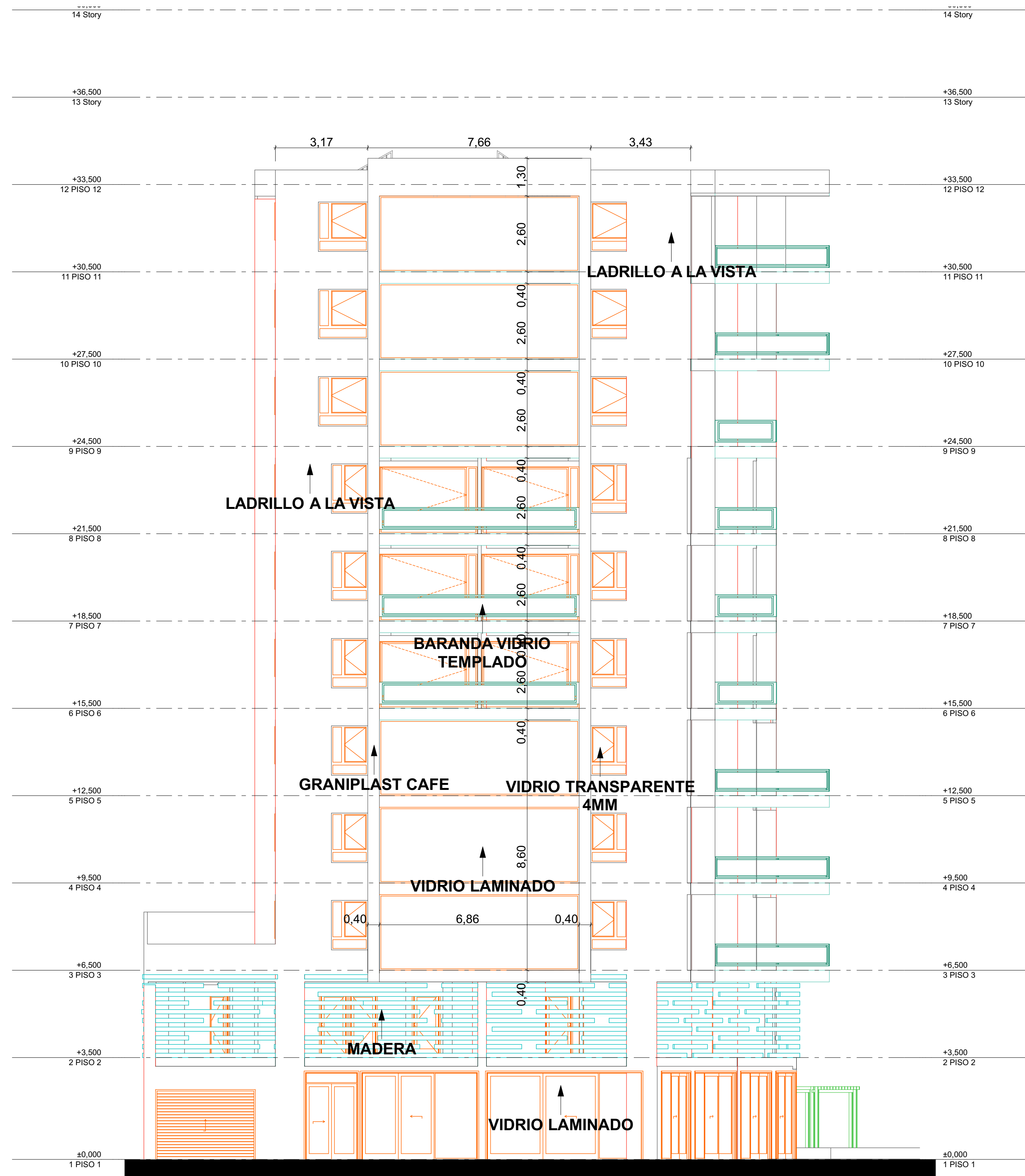
FACHADA SUR
