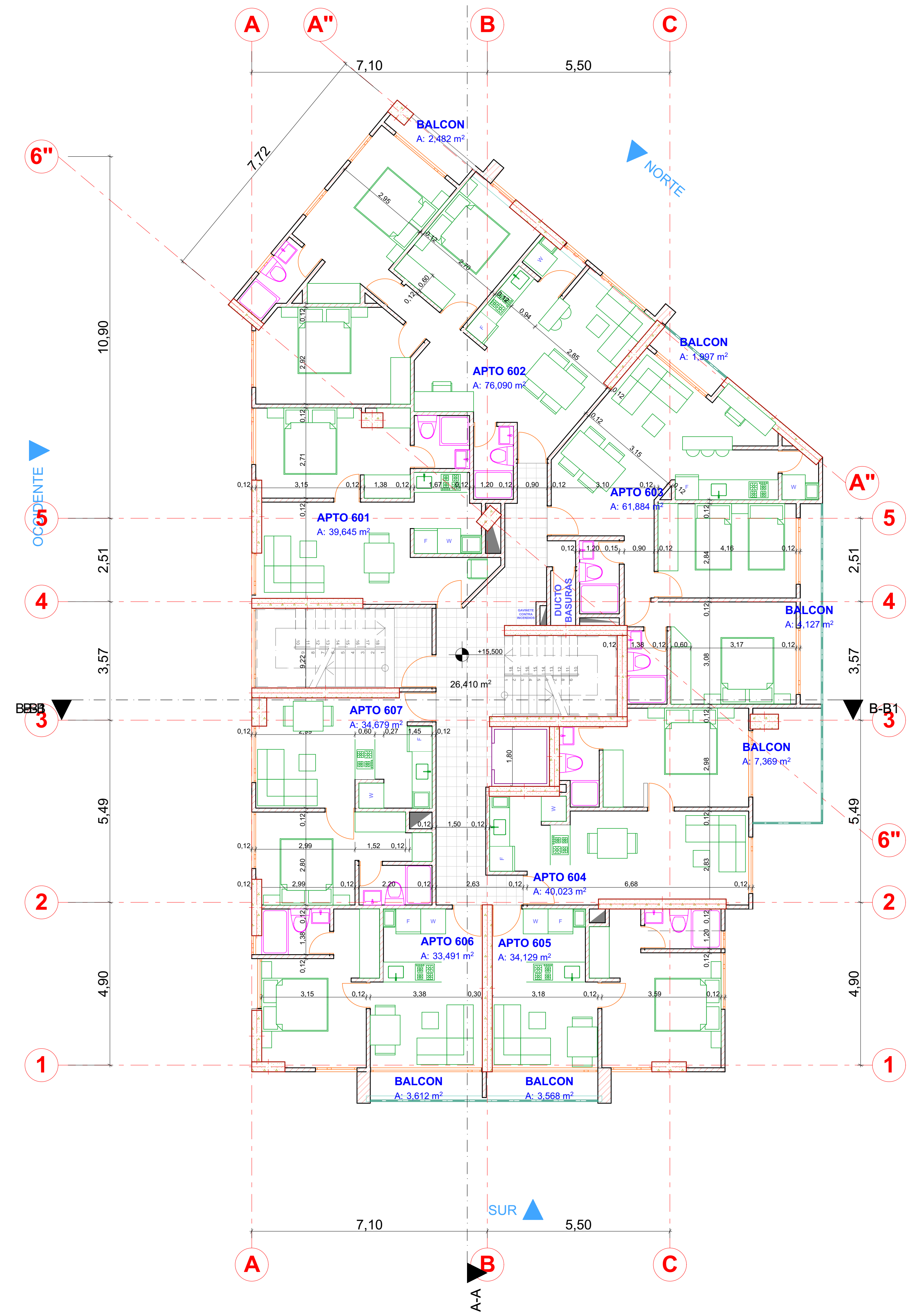
PLANTA TIPO 6, 7 Y 8
