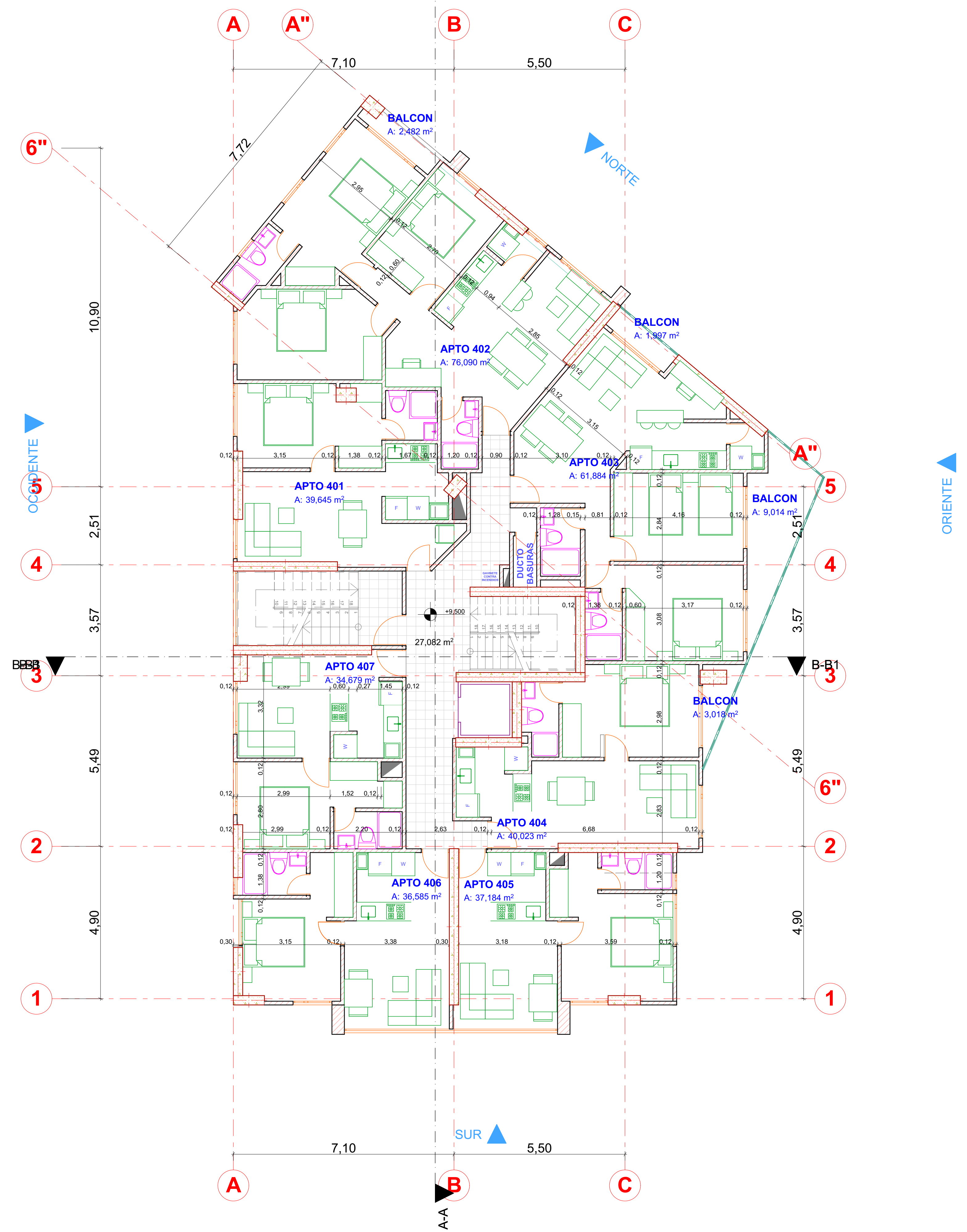
PLANTA TIPO PISOS 4 Y 5
