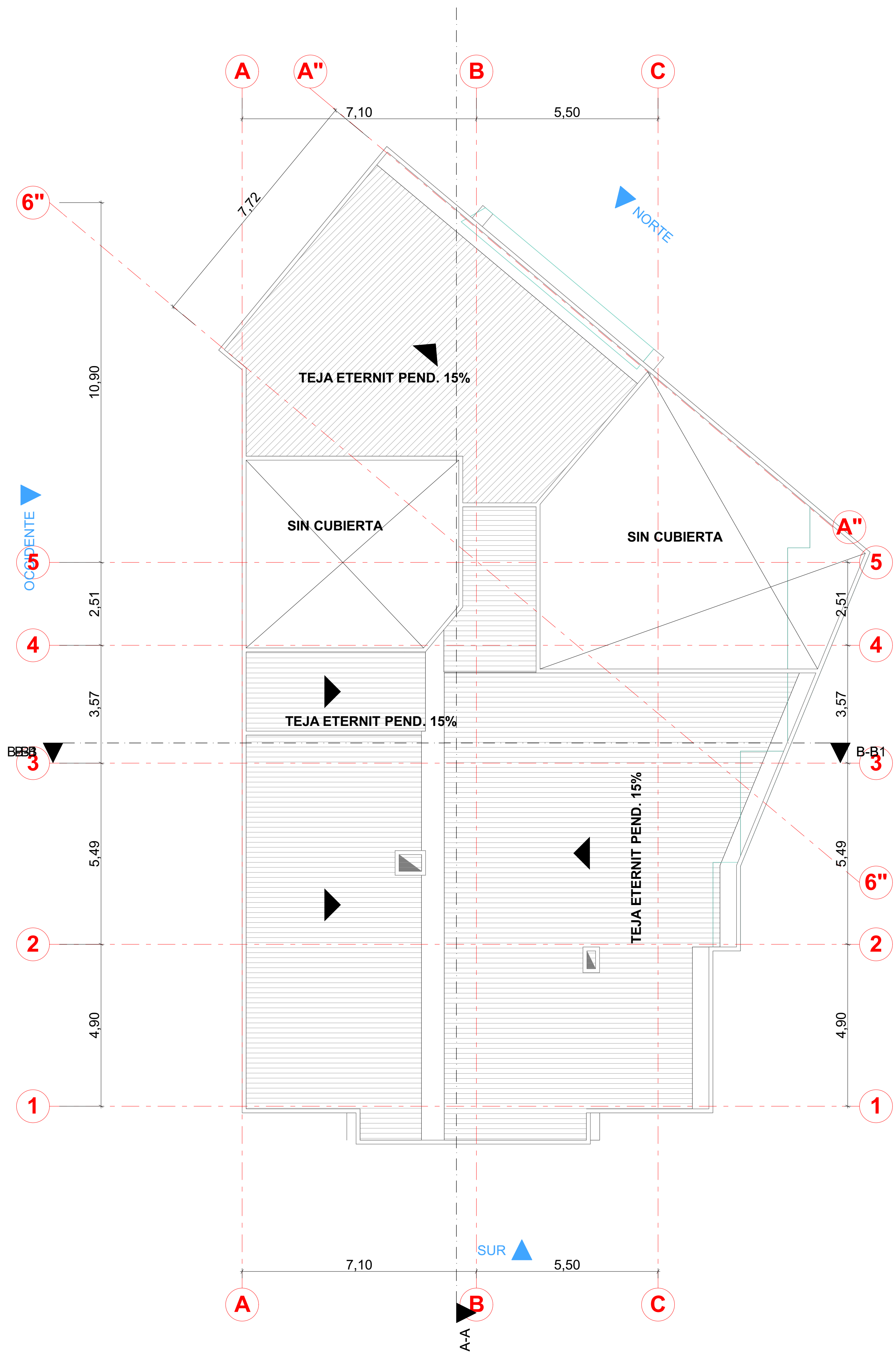
PLANTA PISO 12
