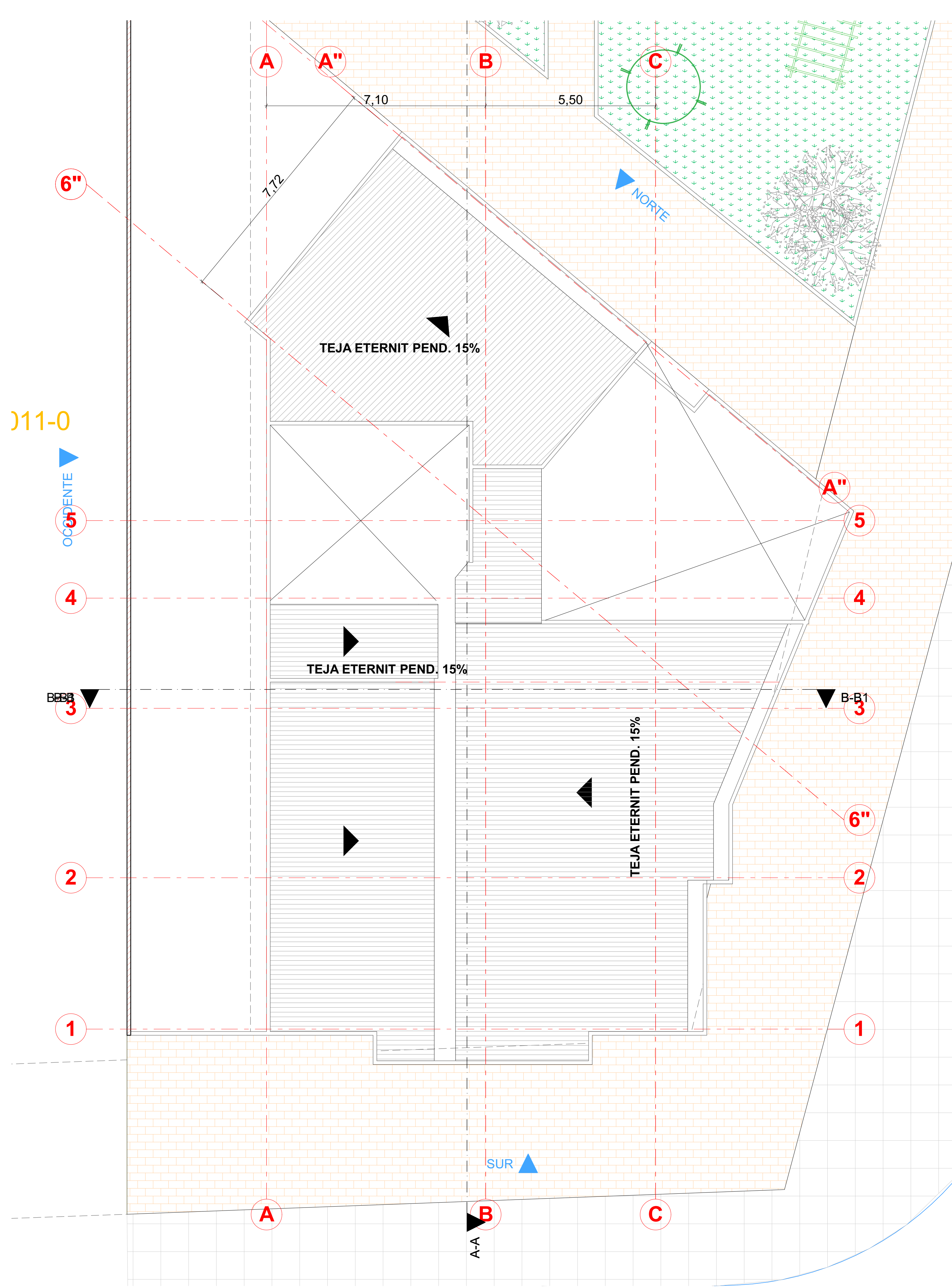
PLANTA CUBIERTAS
