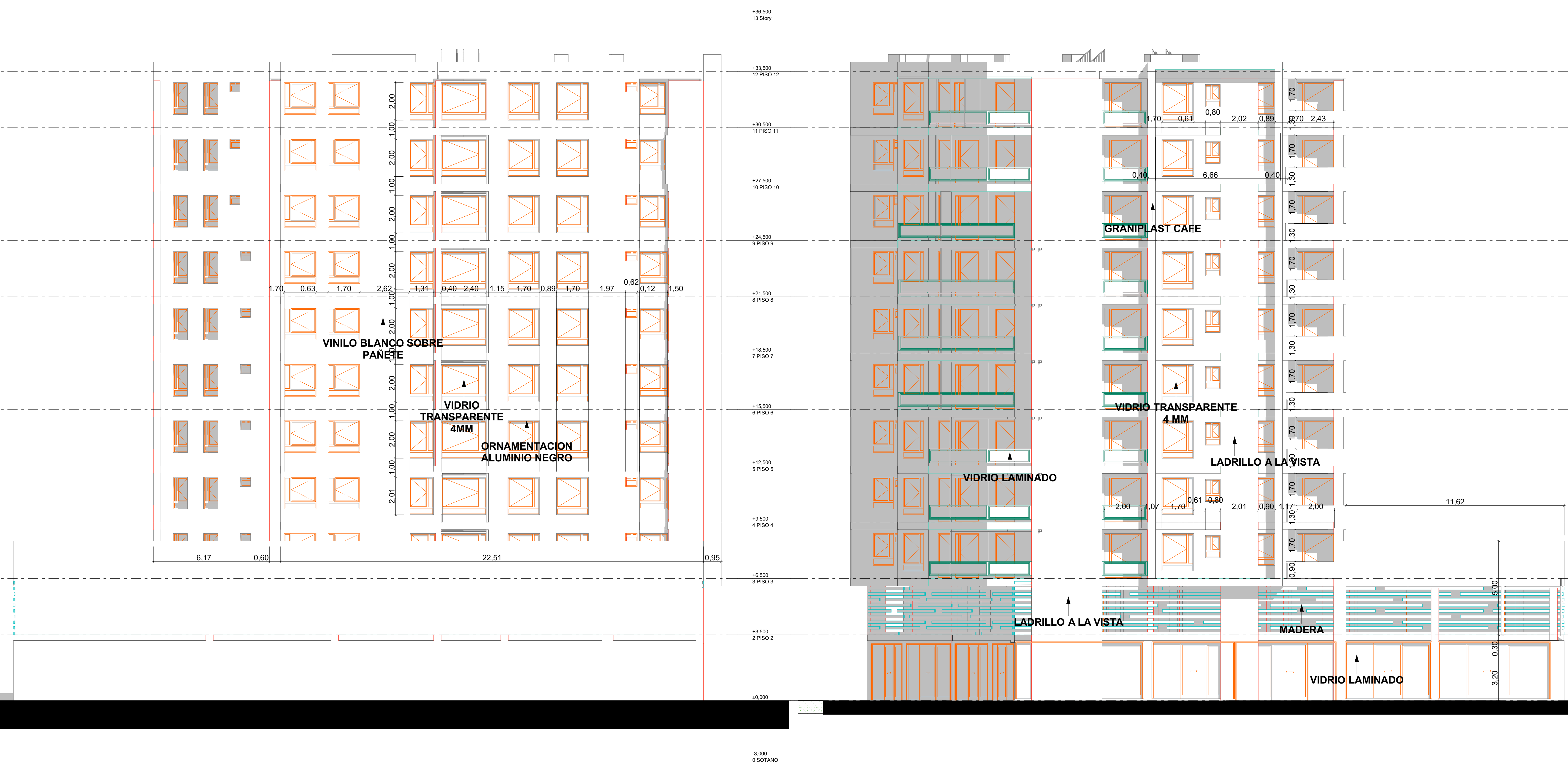
FACHADA OCCIDENTE
