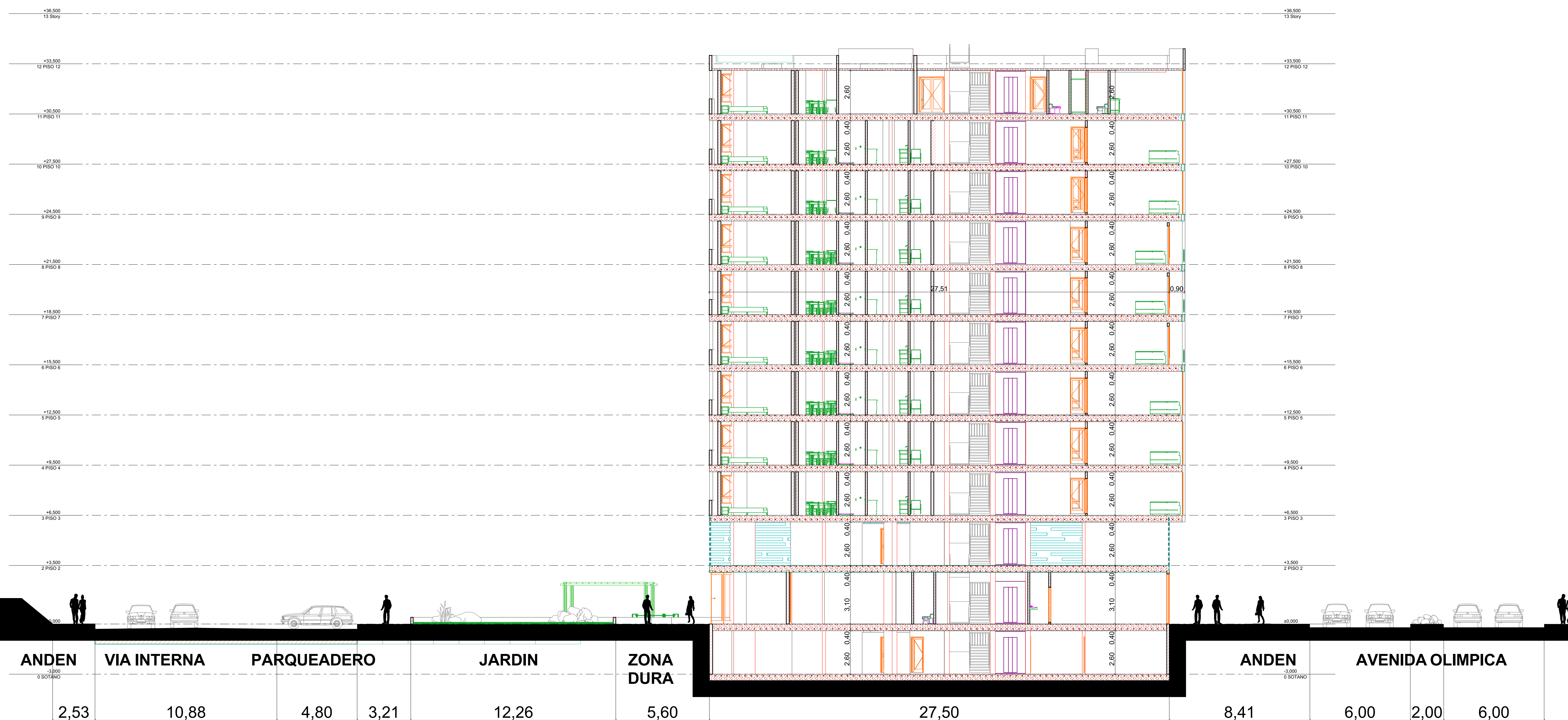
CORTE A-A
