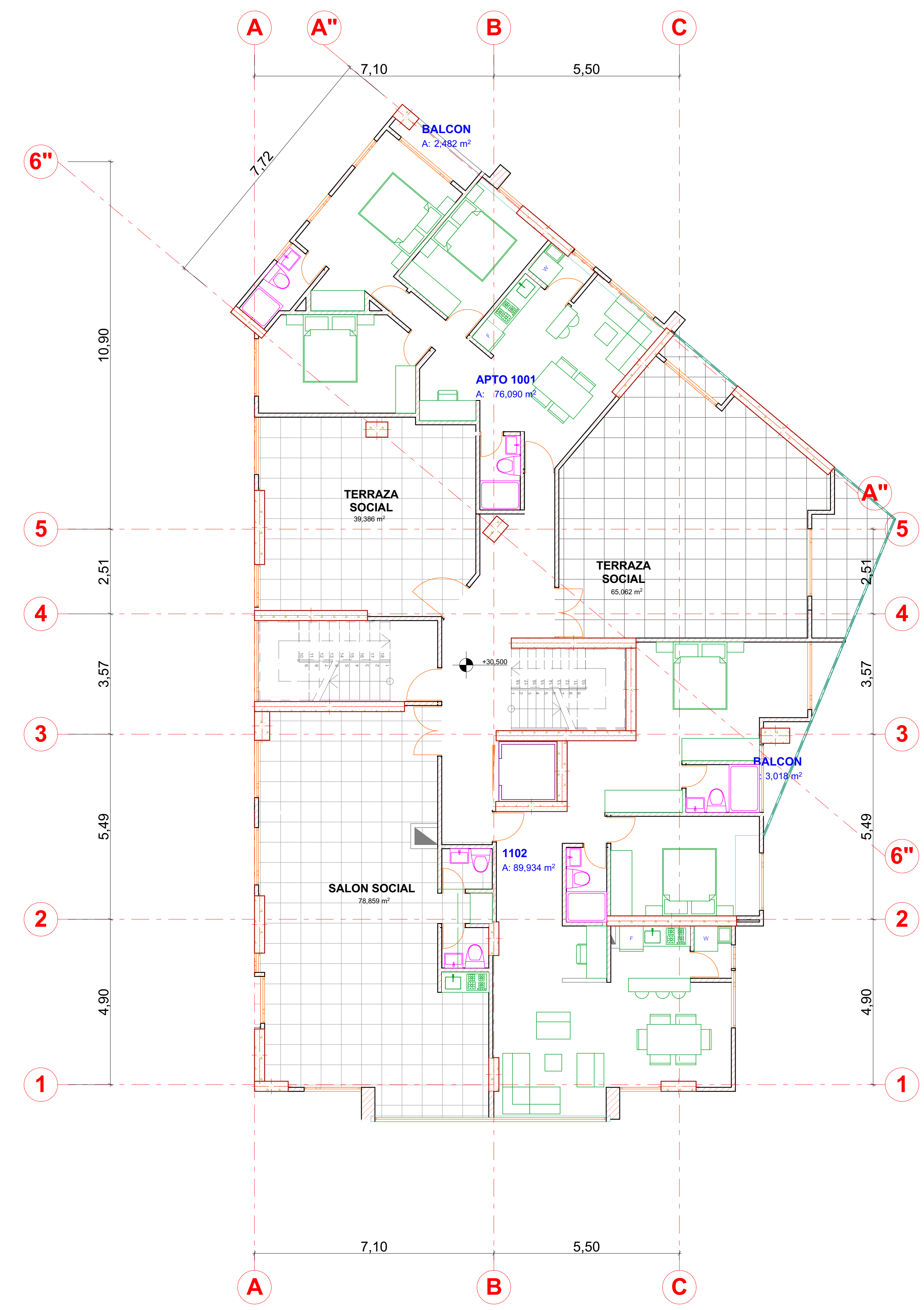
PLANTA PISO 11
