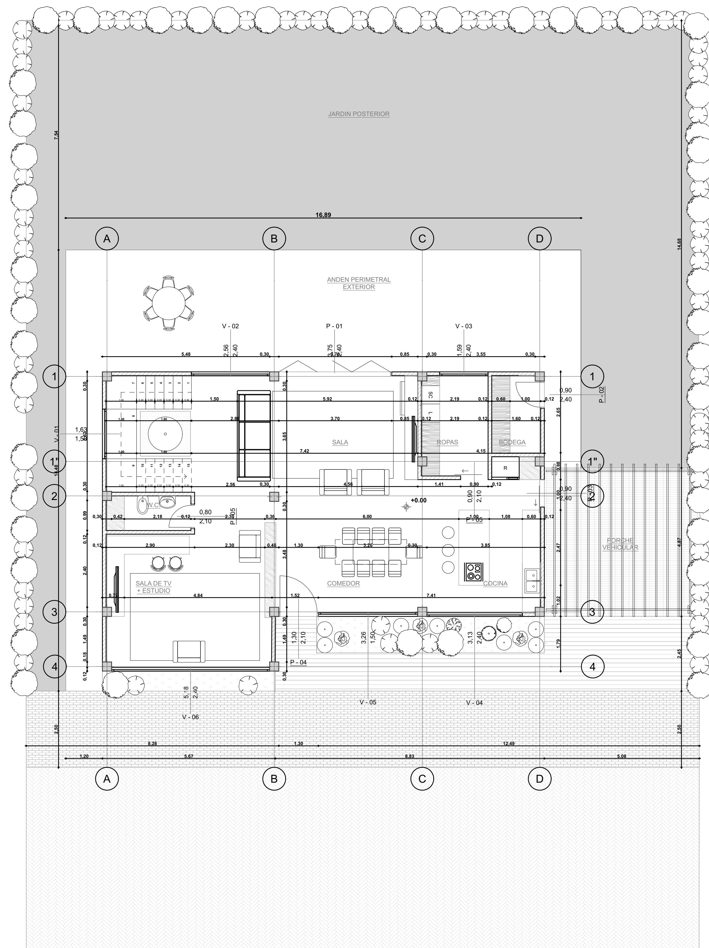
TIPOLOGIA VIVIENDA 2 NIVELES
