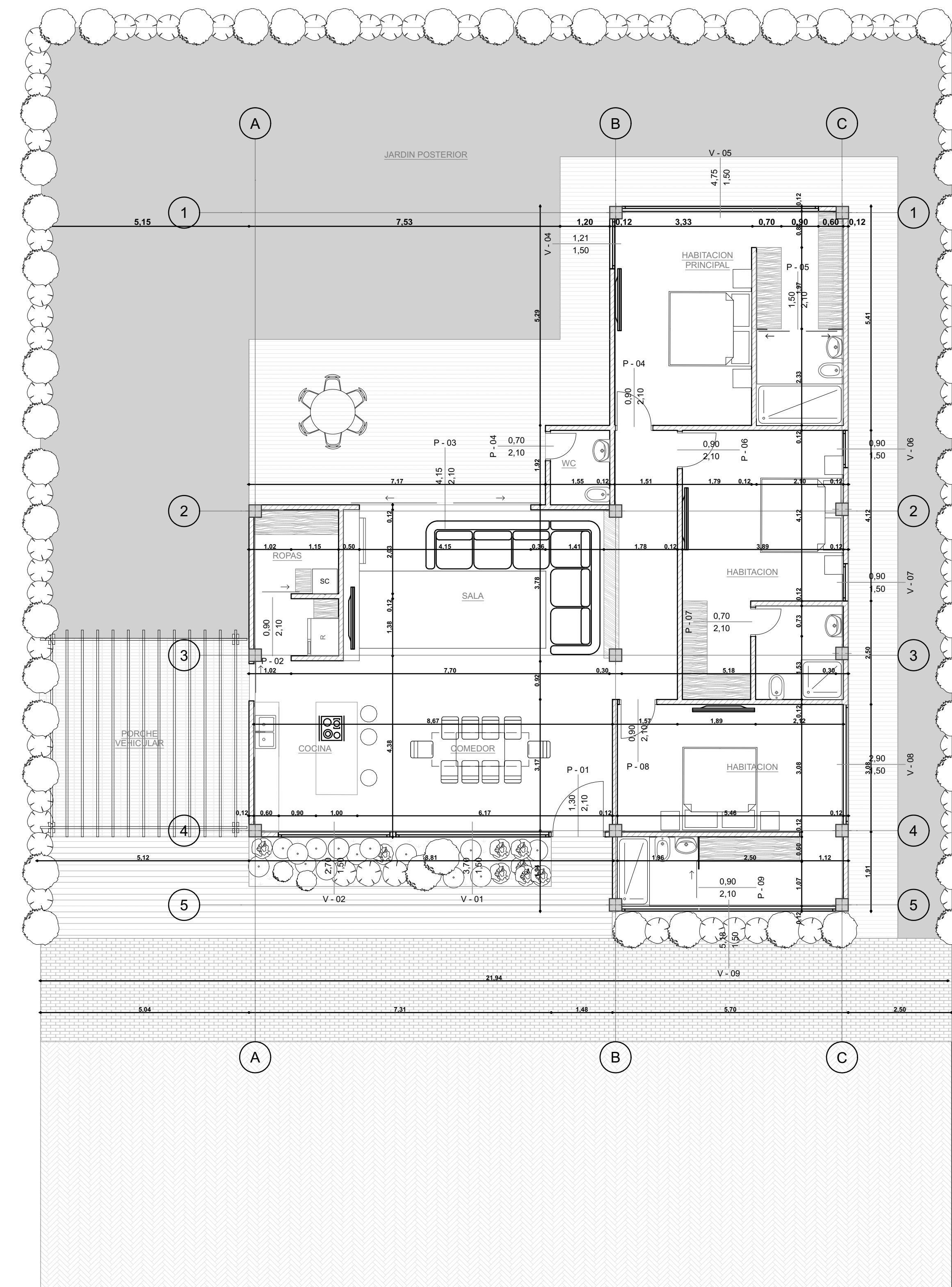
TIPOLOGIA VIVIENDA 1 NIVEL
