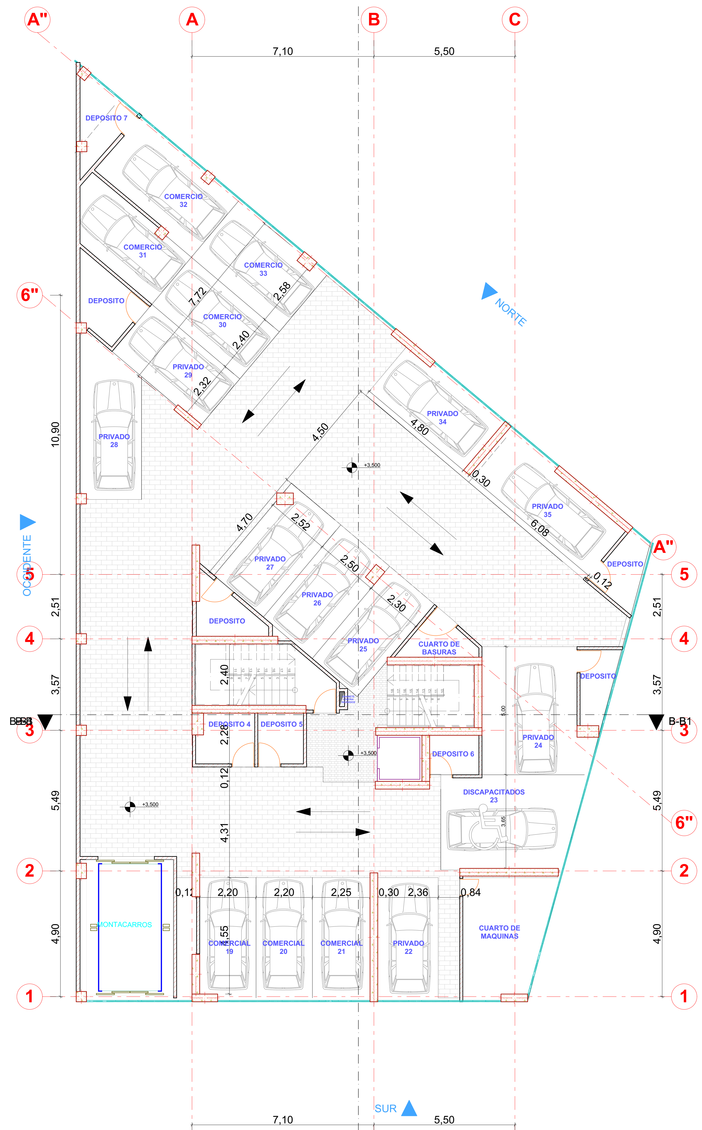
PLANTA PARQUEADEROS SEGUNDO PISO
