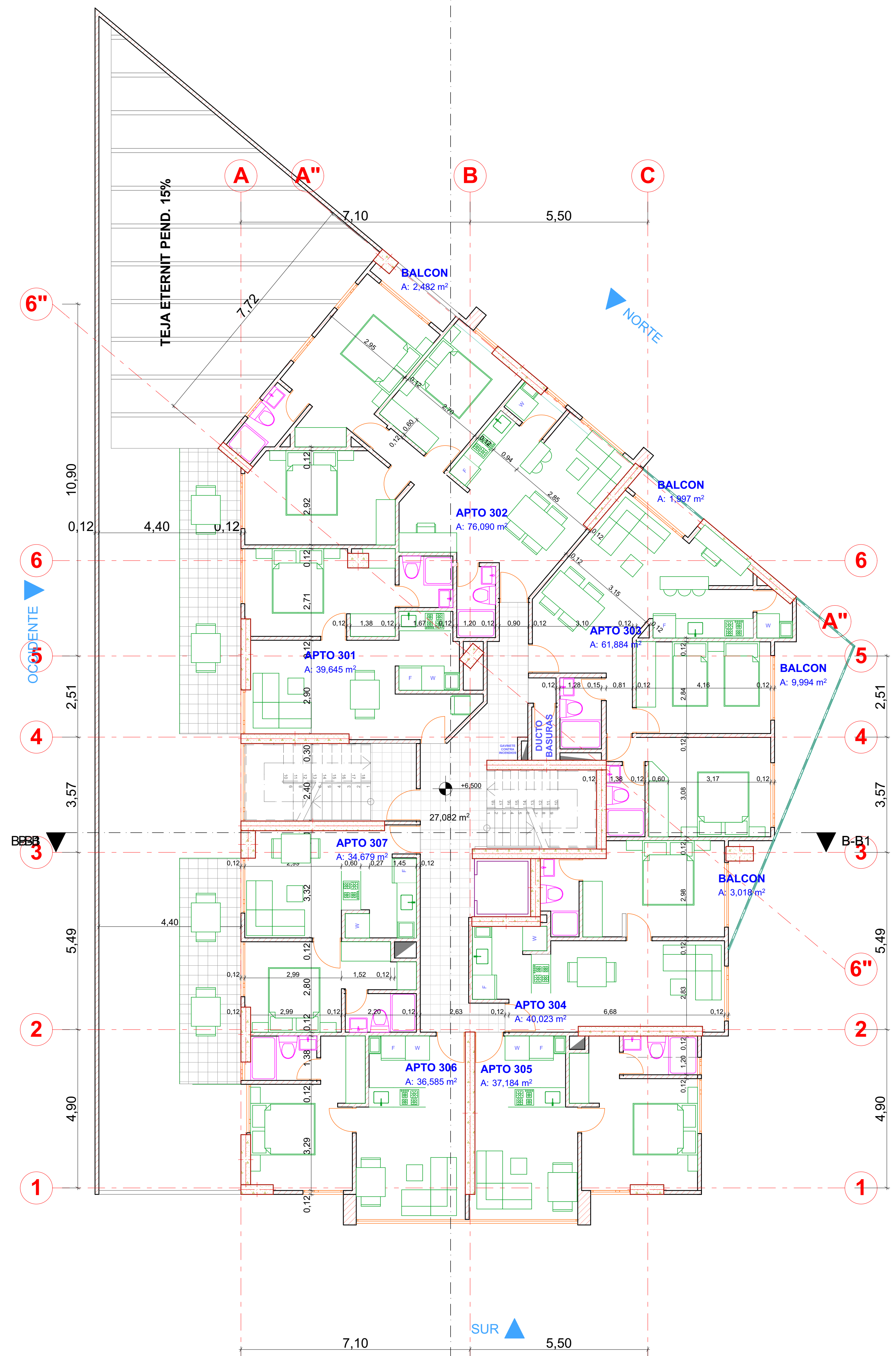
PLANTA APARTAMENTOS 3 PISO
