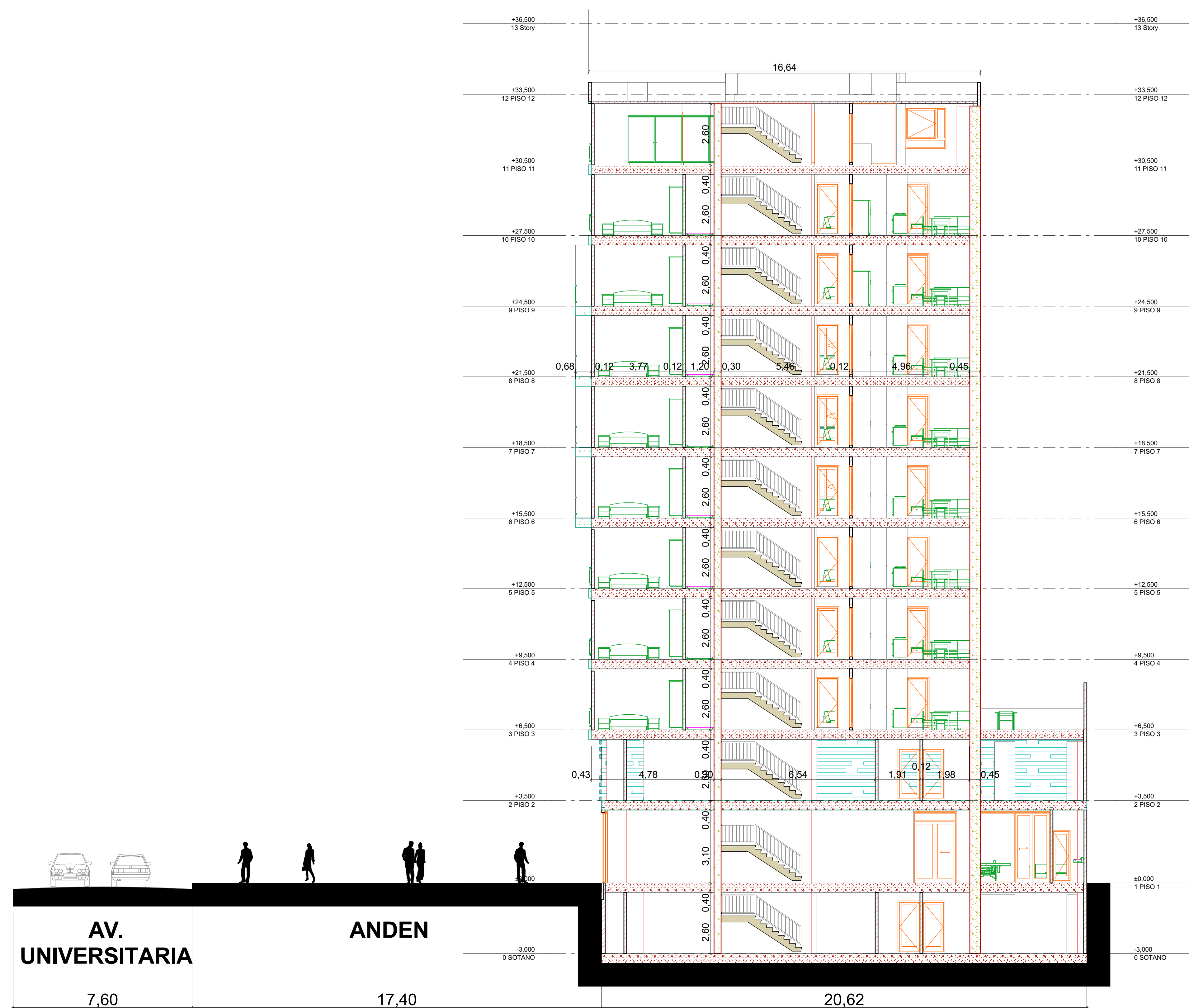
CORTE B-B
